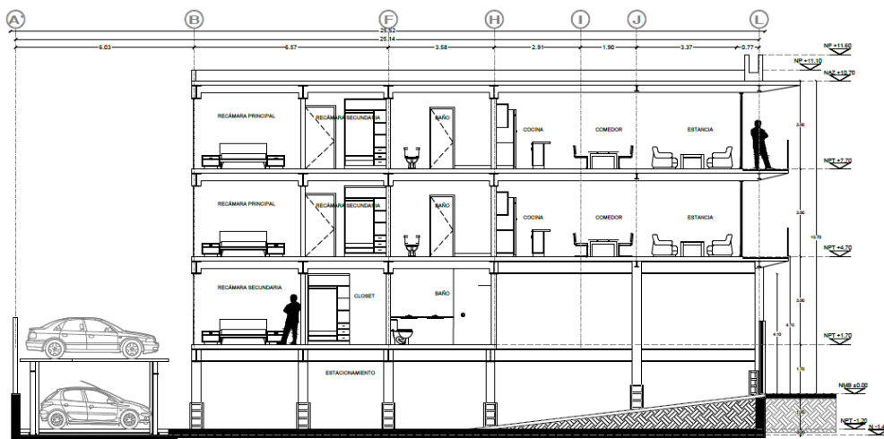
CORTE A-A'
