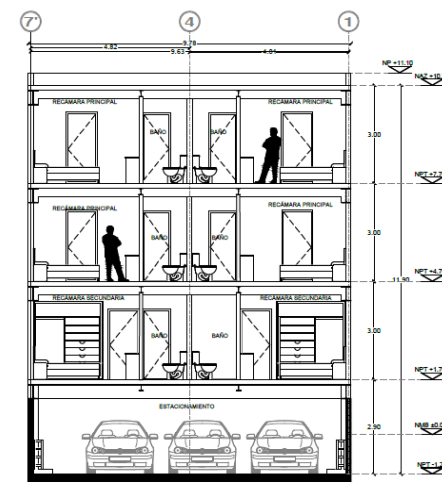
CORTE B-B'
