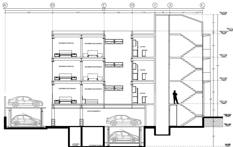
CORTE C-C'
